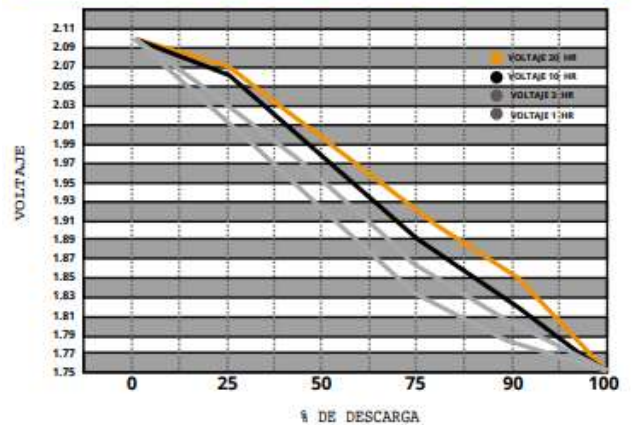
VOLTAJE VS. % DE DESCARGA
