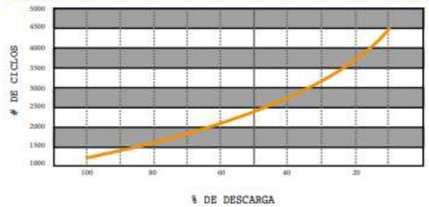
CICLOS DE VIDA V.S. PROFUNDIDAD DE LA DESCARGA
